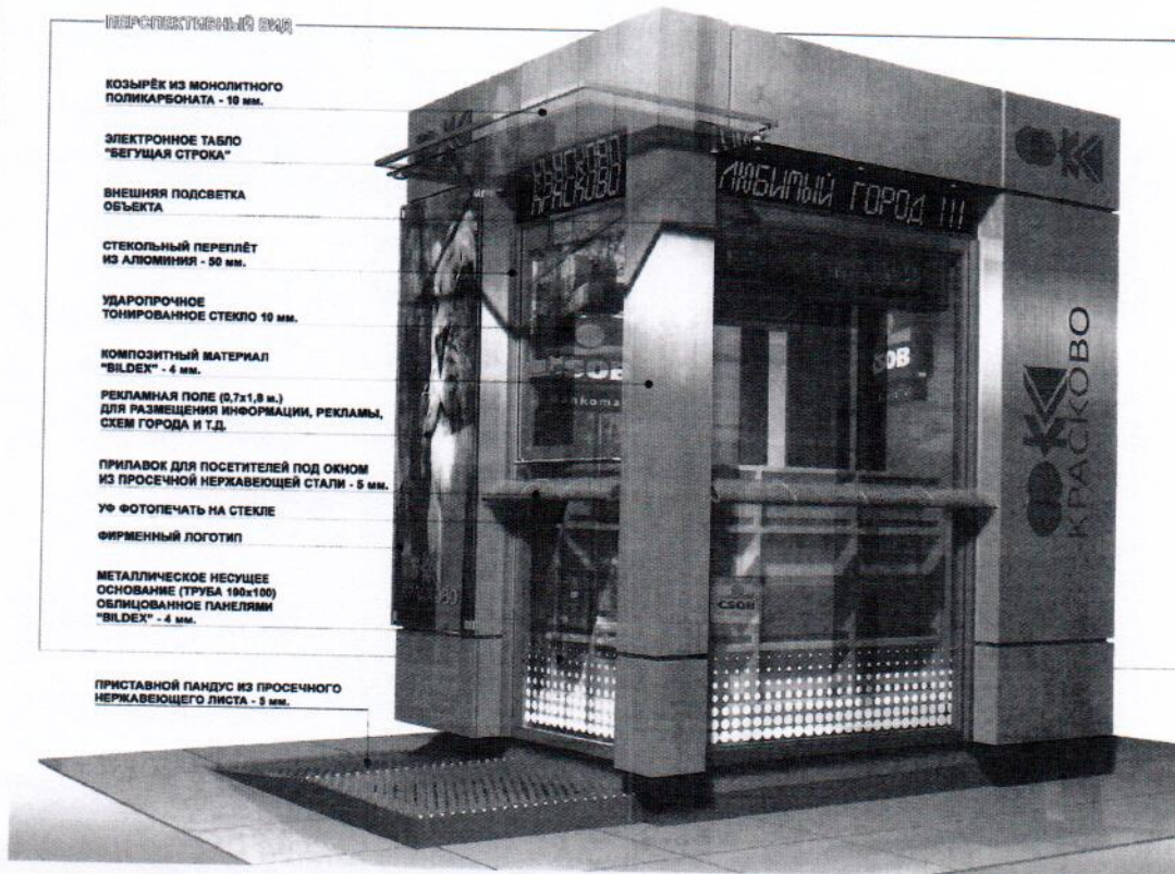
ПЕРСПЕКТИВНЫЙ ВИД
