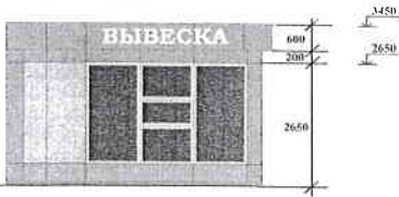
фасад А
